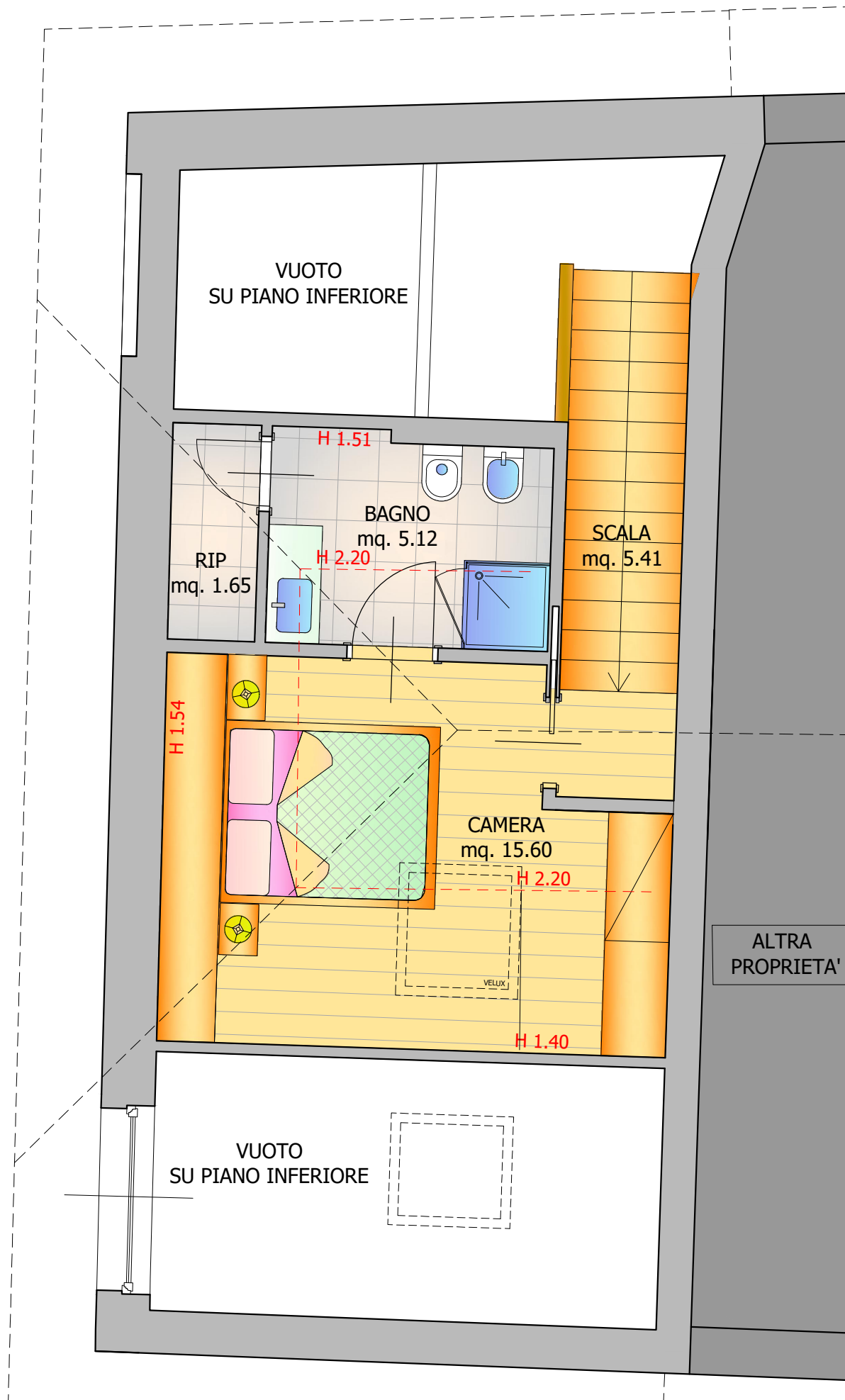
PIANTA PIANO SOPPALCO SCALA 1:50
